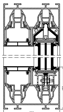
Vodorovný řez Schüco ASS 77 PD.SI Vertical section detail Schüco ASS 77 PD.SI Měřítko 1:8 Scale 1:8
