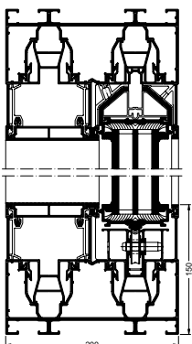
Vodorovný řez Schüco ASS 77 PD.NI Vertical section detail Schüco ASS 77 PD.NI Měřítko 1:8 Scale 1:8
