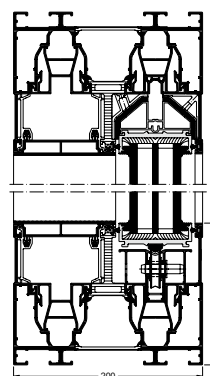
Vodorovný řez Schüco ASS 77 PD.HI Vertical section detail Schüco ASS 77 PD.HI Měřítko 1:8 Scale 1:8
